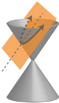
Parabola
