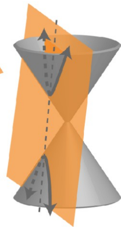
Hyperbola
